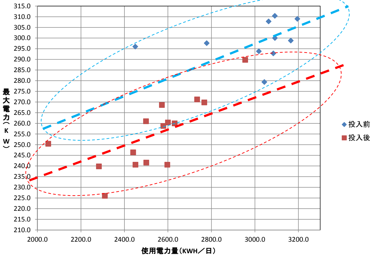
積算電力系計による使用電力量(kWh/日)対最大電力(kW)(M金属加工工場)
