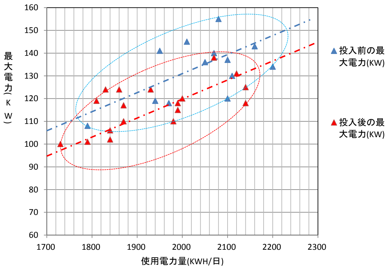
300KVAトランスの使用電力量(KWH/日)に対する最大電力(KW)の 推移(S金属加工事業所)
